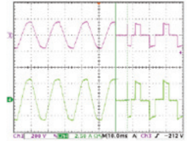
图 7: Off-Line UPS 转换时间
