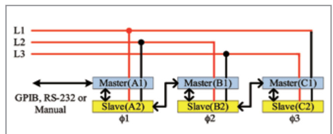
图12: 并联三相Δ接法
