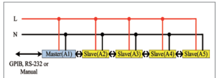
图10: 并联接法
