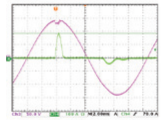
图6: 浪涌电流模式
